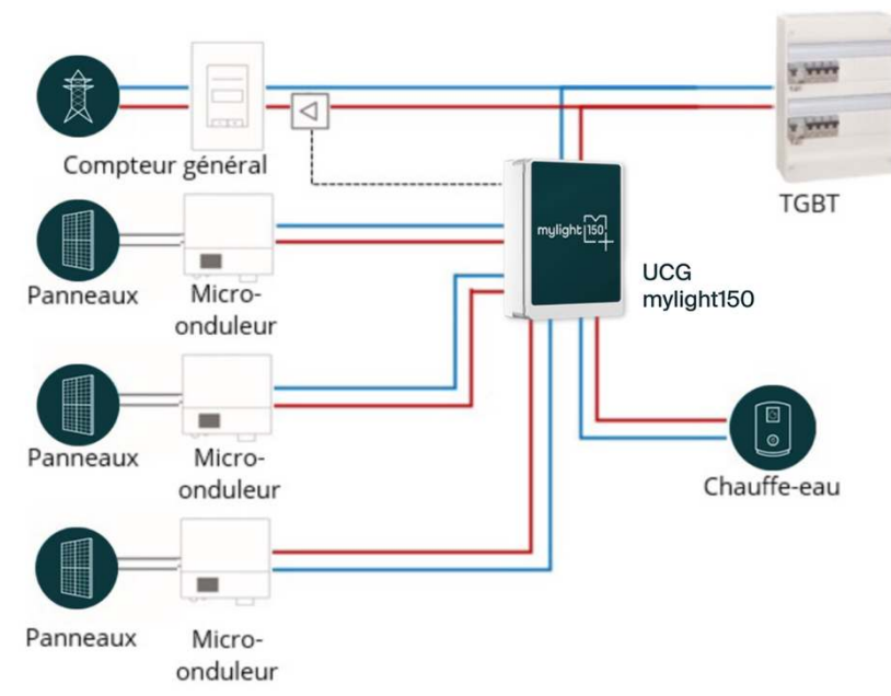
Figure 7. Cas d'utilisation typique et mise en armoire UCG-E3301-11-FR
