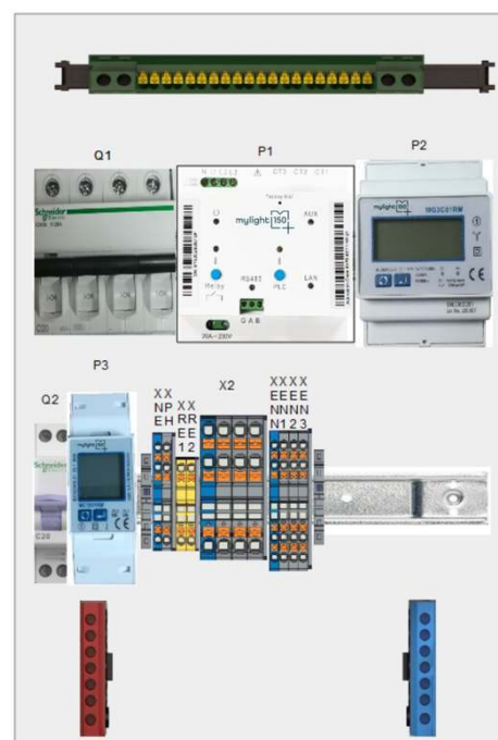
Figure 12. Cas d'utilisation typique et mise en armoire UCG-X0302-31-FR
