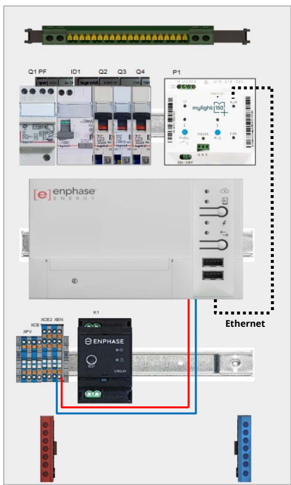
Figure 31. Schéma de principe de montage de la passerelle Envy
