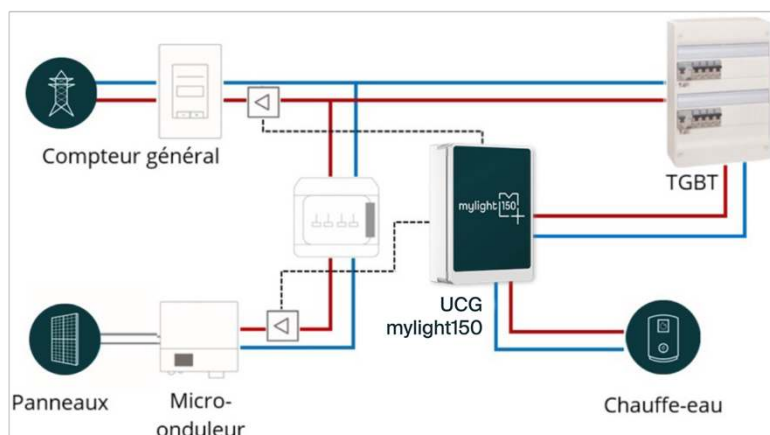
Figure 11. Cas d'utilisation typique et mise en armoire UCG-X0301-11-FR
