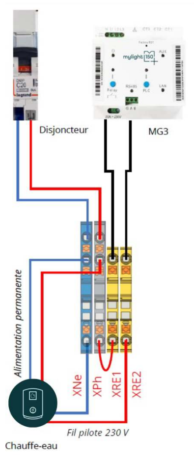
Figure 25. Schéma de pilotage d'un chauffe-eau thermodynamique monophasé avec un pilotage 230V
