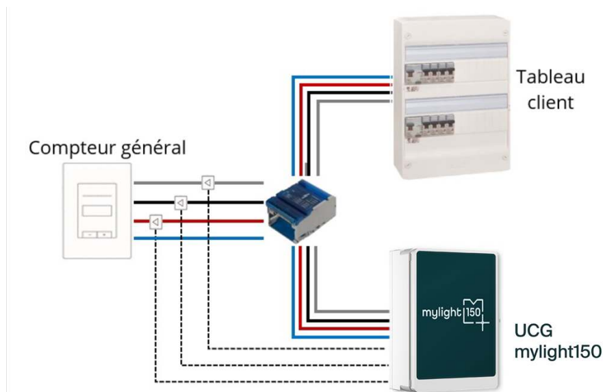
Figure 29. Positionnement des TC dans le cadre d'une installation triphasée.
