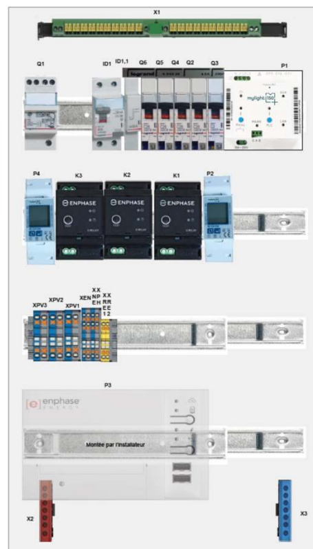
Figure 7. Cas d'utilisation typique et mise en armoire UCG-E3301-11-FR
