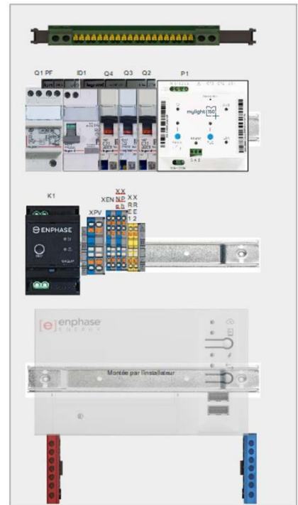
Figure 5. Cas d'utilisation typique et mise en armoire UCG-E4301-11-FR
