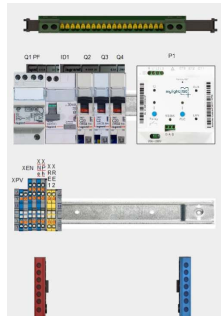
Figure 1. Cas d'utilisation typique et mise en armoire UCG-U4301-11-FR et UCG-U6301-11-FR
