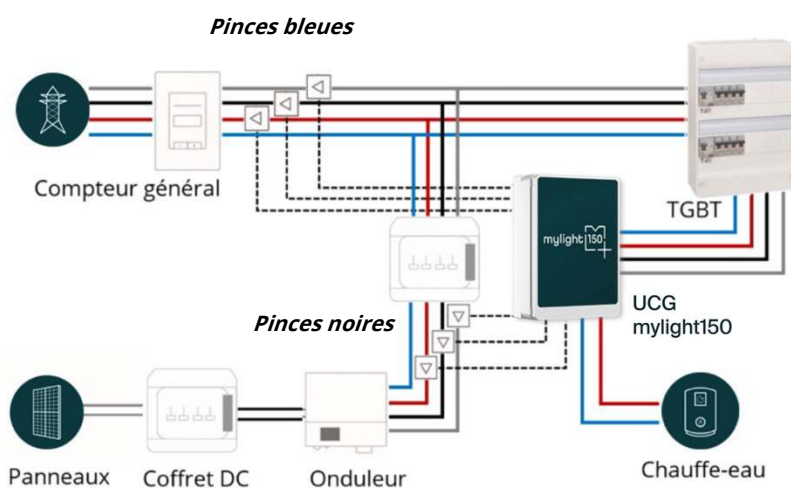
Figure 12. Cas d'utilisation typique et mise en armoire UCG-X0302-31-FR
